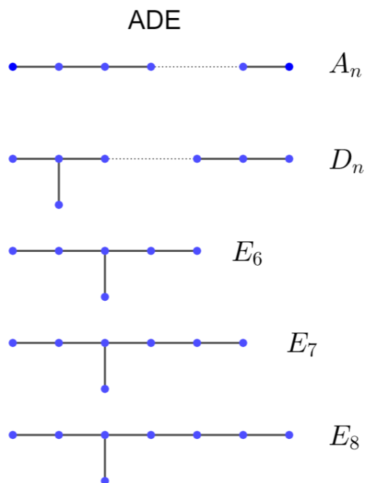
Figura 14: Grafos ADE de Dynkin
